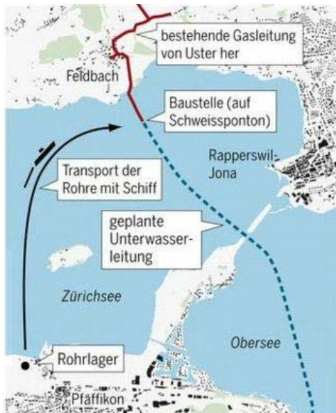
Neue Gasleitung (Bild: TA-Grafik mt)
